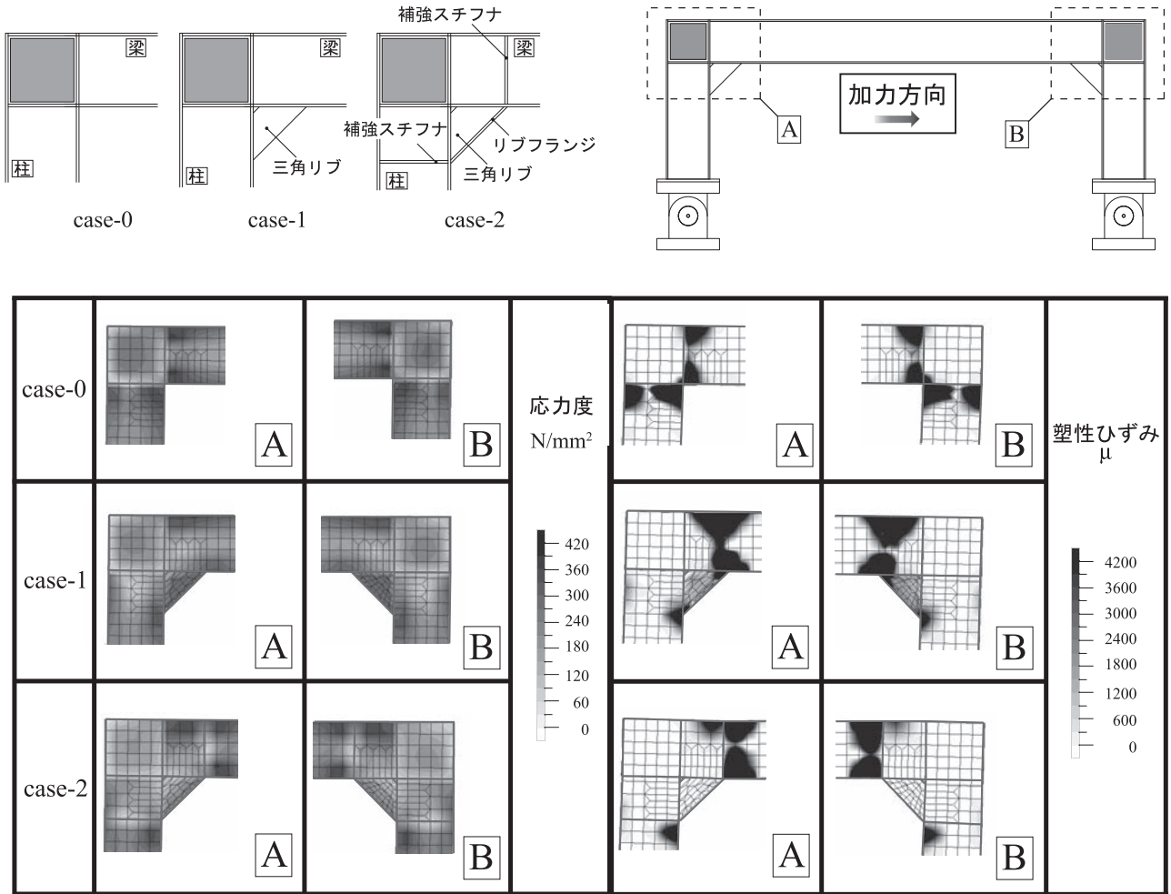
図10 降伏時の応力分布 (i) と終局時の塑性ひずみ分布 (ii)
