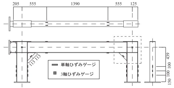
図5 ゲージ計測位置
