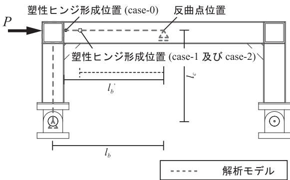
図6 試験体形状とモデル
