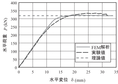
図7 P-δ関係
