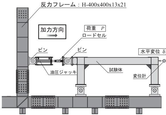
図4 実験装置
