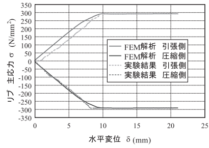
図8 リブσ-δ関係
