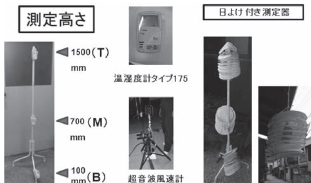
資料3. 測定器, 測定高さ
