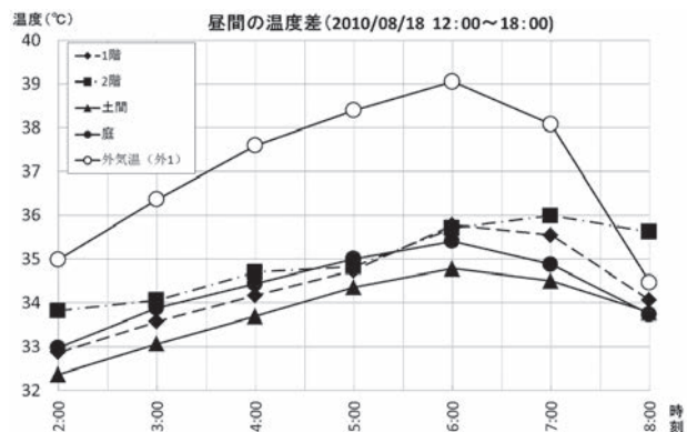
図5. 気温の時間変化（12時～18時）
