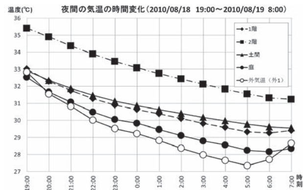
図4. 気温の時間変化（19時～翌日8時）
